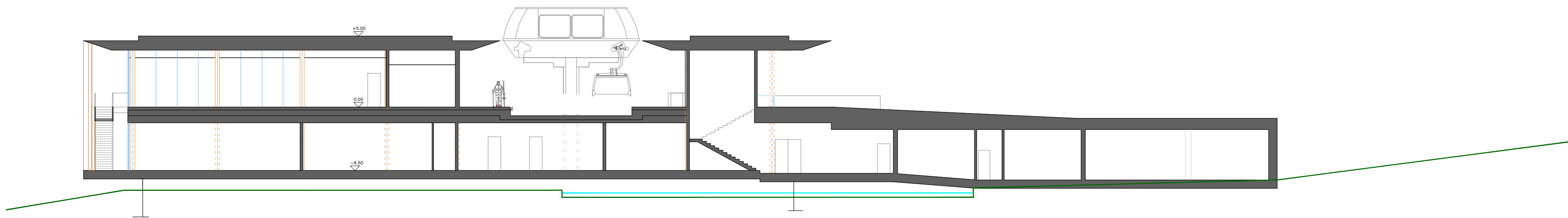
SEZIONE 33
