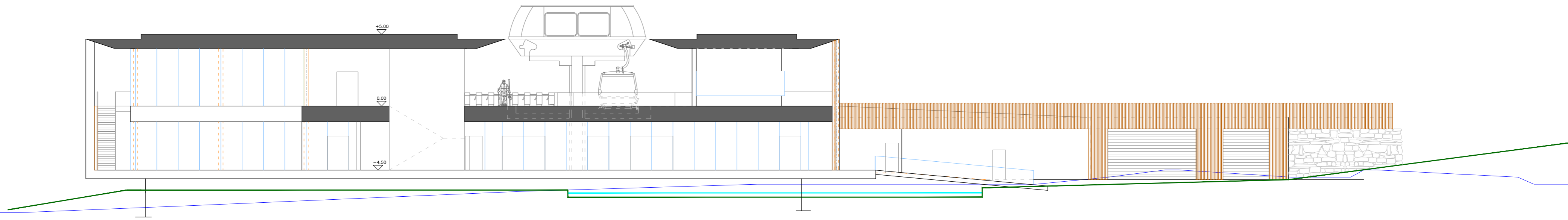
SEZIONE 11
